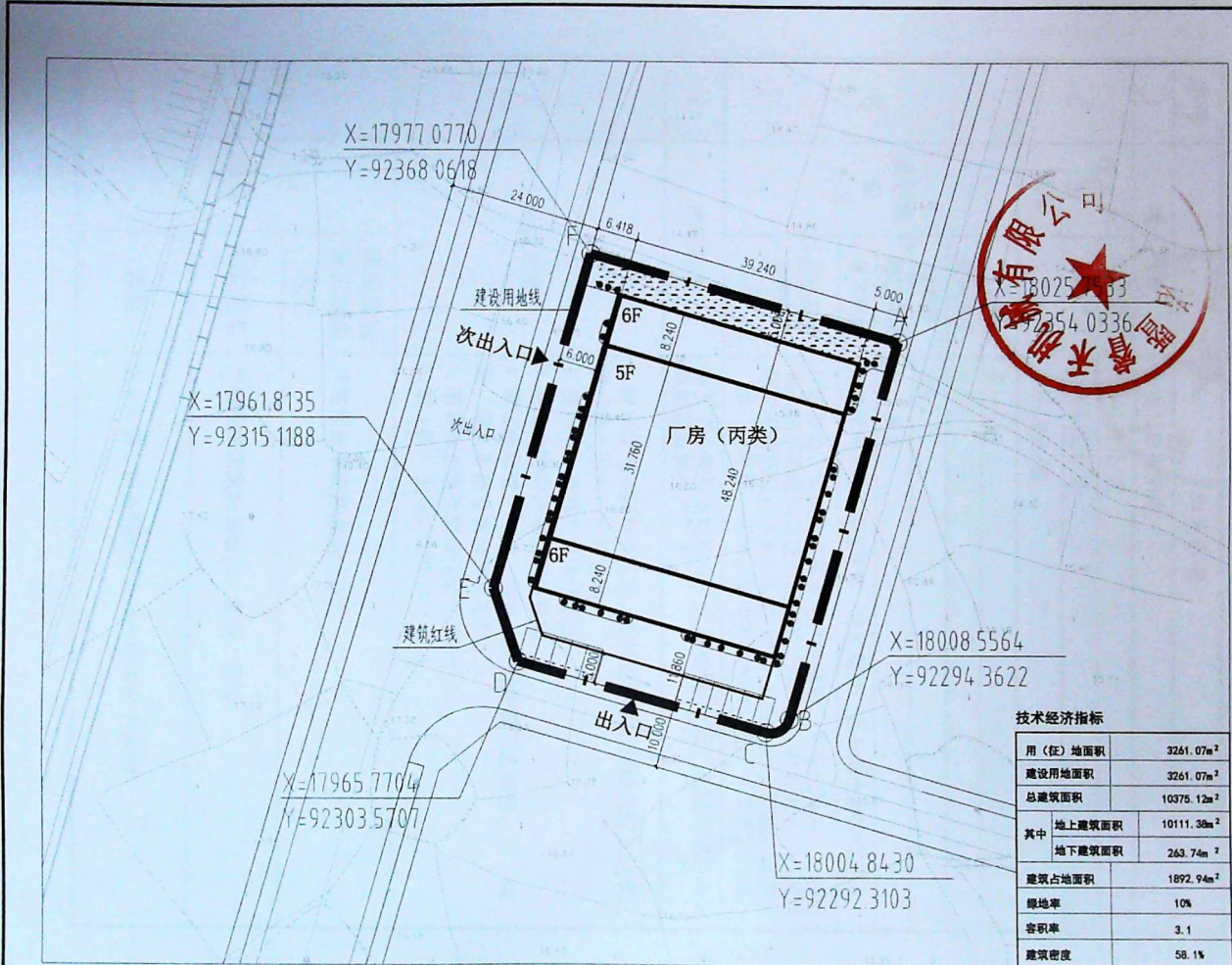
总平面布置图 1:500
